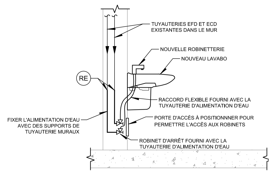
POSITIONNEMENT ROBINETS
