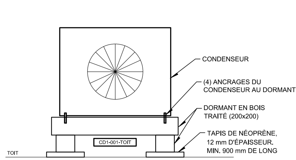
INSTALLATION DE LA BASE D'UN CONDENSEUR AU TOIT
