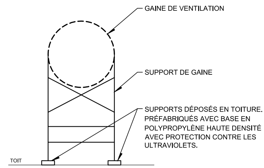
SUPPORTS DÉPOSÉS EN TOITURE POUR UNE GAINÉ DE VENTILATION
