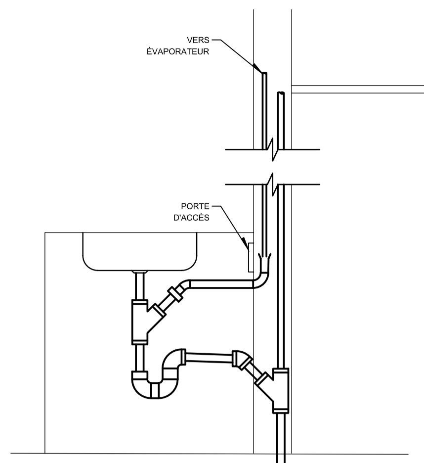
DRAINAGE INDIRECT - UNITÉ DE CLIMATISATION (ÉVAPORATEUR) SUR L'ÉVIER
