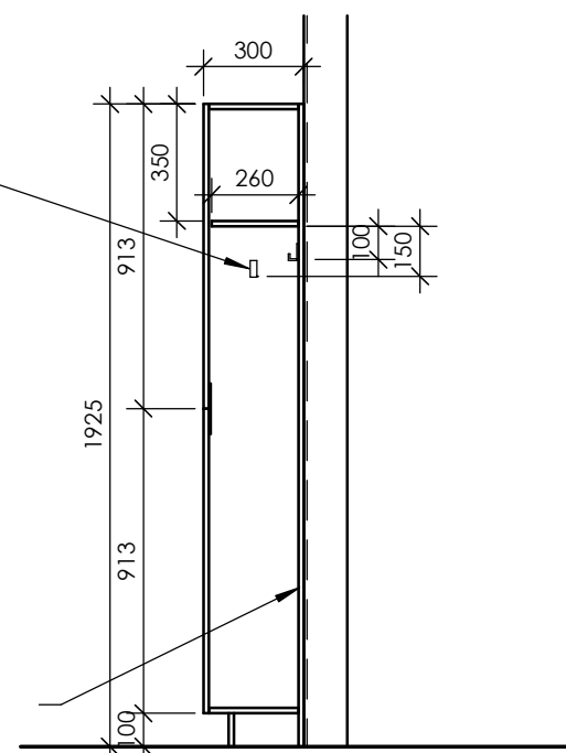
3 A801 DÉTAIL EN COUPE VESTIAIRES ÉDUCATRICES 1 : 25
