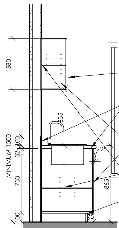
2 CUISINETTE - COUPE A805 1 : 25
