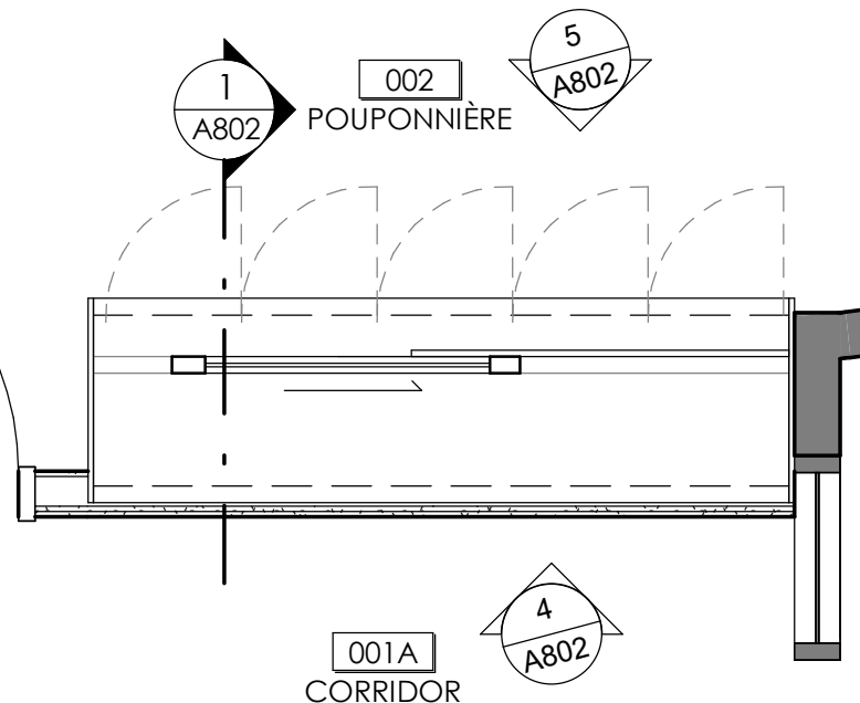
2 PASSE POUPONS - PLAN 1 A802 1 : 25
