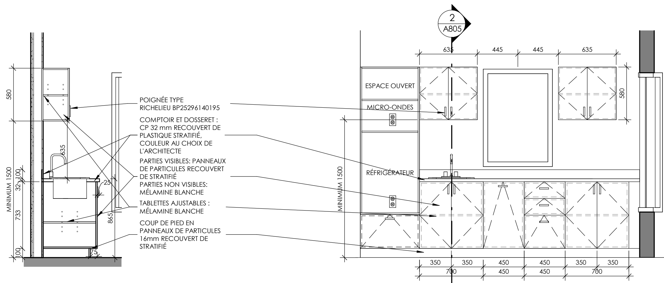
3 CUISINETTE - ÉLEVATION A805 1 : 25
