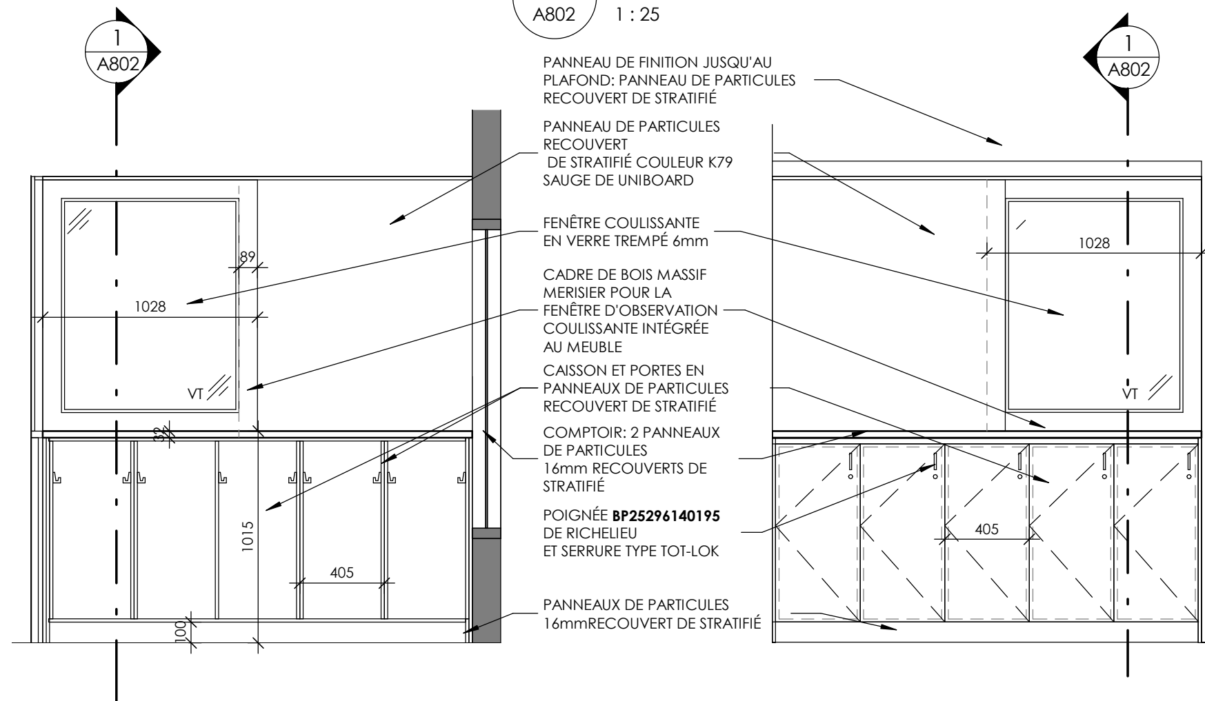
4 PASSE-POUPONS - ÉLÉVATION CÔTÉ CORRIDOR A802 1 : 25
