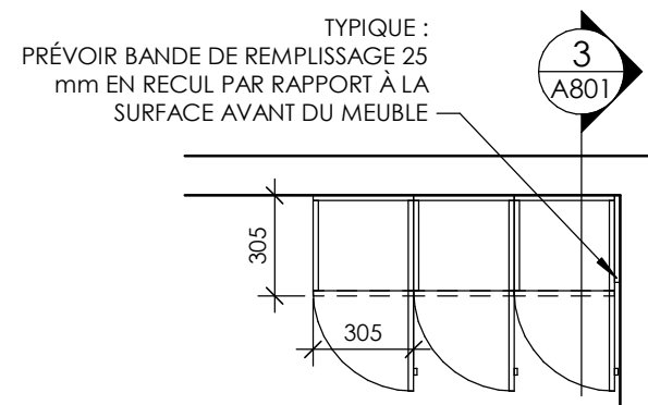
1 A801 DÉTAIL EN PLAN VESTIAIRES ÉDUCATRICES 1 : 25
